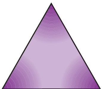
Acutángulo 3 ángulos agudos
