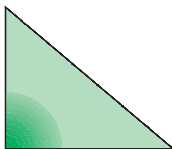
Rectángulo 1 ángulo recto
