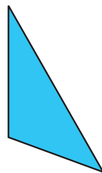
Escaleno 3 lados desiguales
