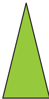
Isósceles 2 lados iguales
