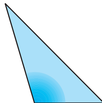
Obtusángulo 1 ángulo obtuso
